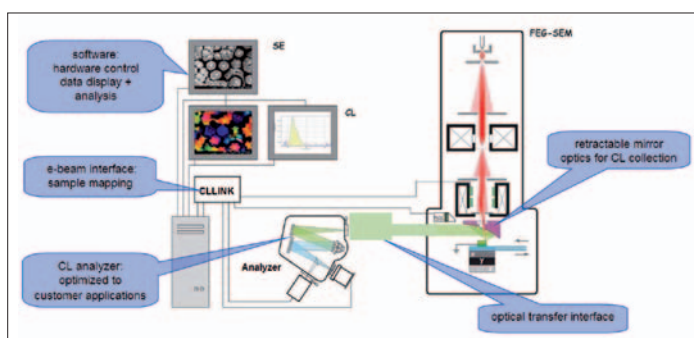
HCLUE-KL-Systemaufbau
